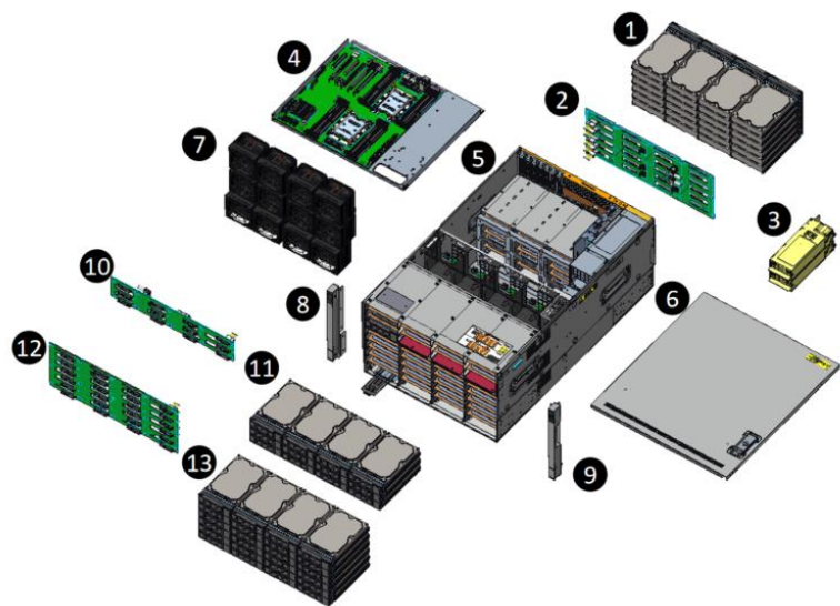
结构图 1-3
