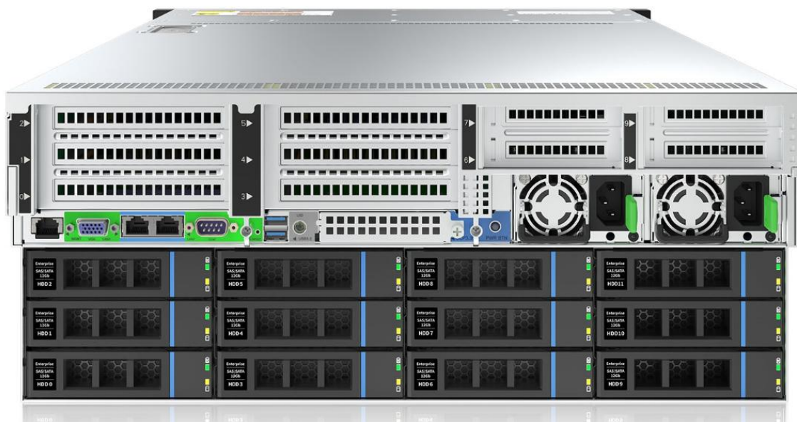
36 盘后视图 1-3
