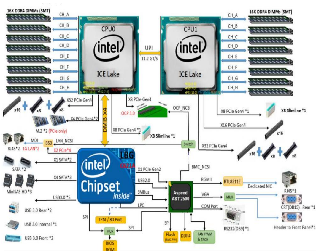
主板逻辑框图 1-4
