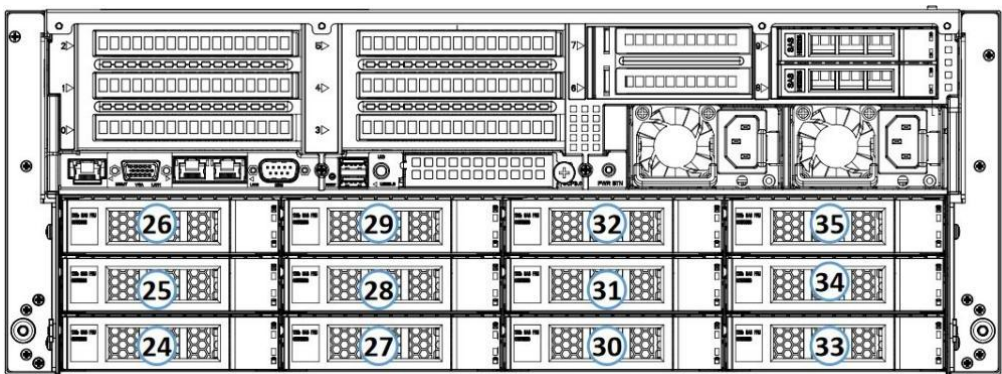
后置 12 盘位图 2-13
