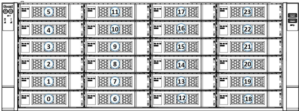
前置 24 盘位图 2-12
